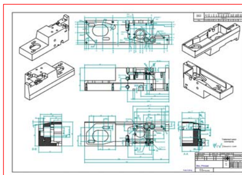
Plans mécaniques - Détail d'usinage -
