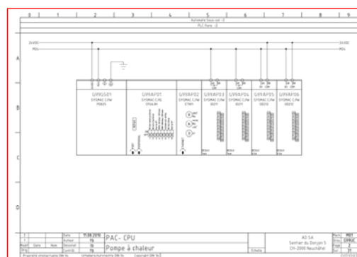
Schémas électriques
